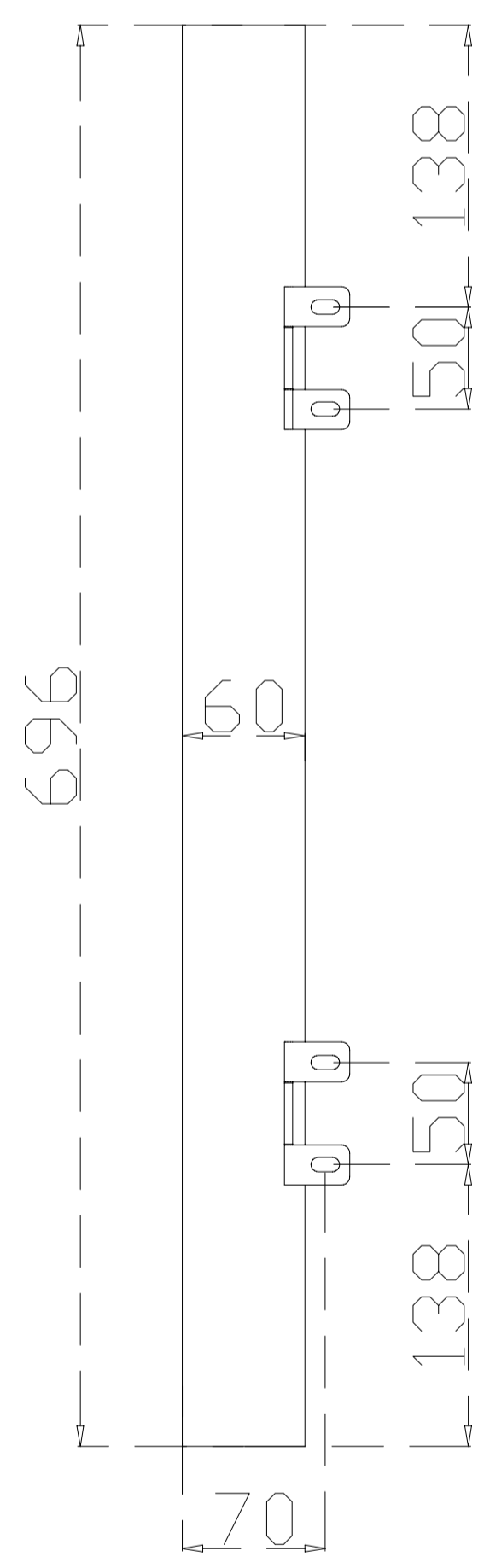
MQ 7907 * 700 mm
