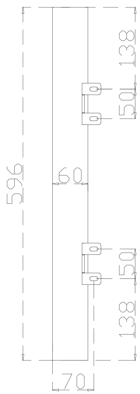
MQ 7906 * 600 mm
